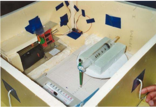
Mesure de pression par seringue
