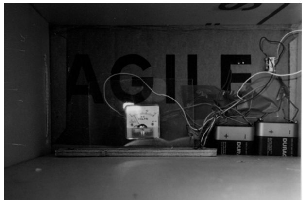
Photographie en vol d'un voltmètre relié à une thermistance placée à l'extérieur
